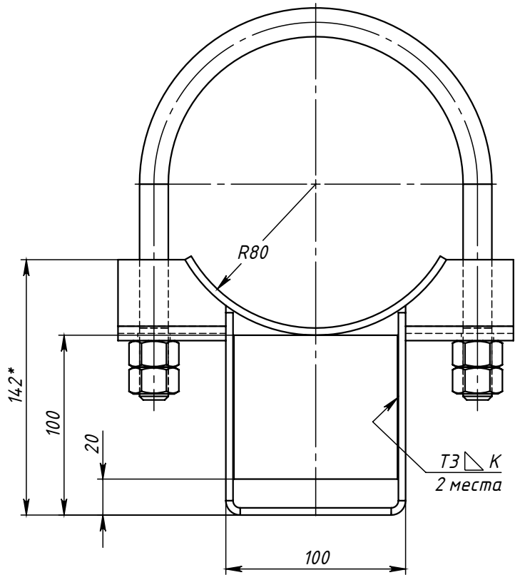
Поз.2 (Ложемент)
