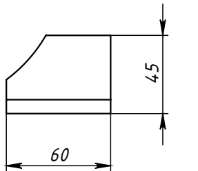
Поз.4 (Ушко)
