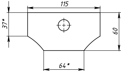
Поз.4 (Ушко) развертка
