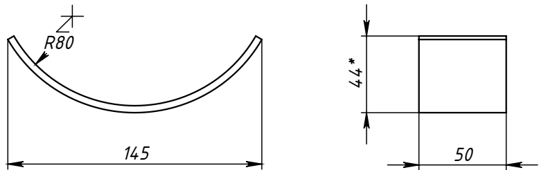
Поз.2 (Ложемент)
